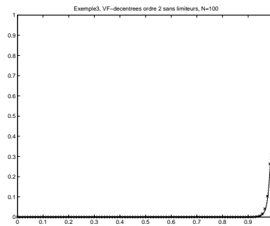
Figure 19: Exemple 3, VF-d/ ordre 2/sans limiteurs, N=100, x =solution approchée
