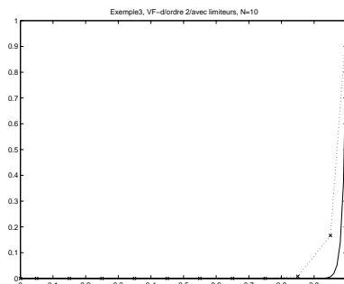
Figure 22: Exemple 3, VF-d/ordre 2/avec limiteurs, N=10, x=solution approchée
