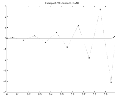
Figure 8: Exemple 3, VF-c, N=10, x =solution approchée
