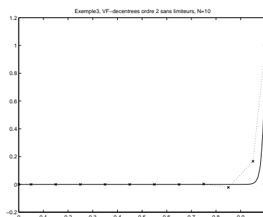
Figure 17: Exemple 3, VF-d/ordre 2/sans limiteurs, N=10, x=solution approchée
