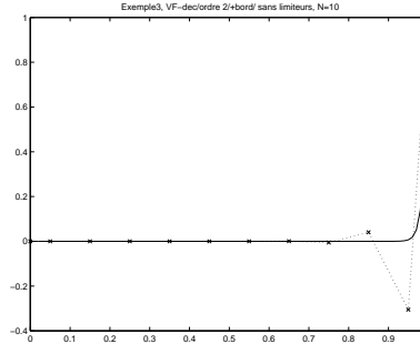
Figure 20: Exemple 3, VF-d/ordre 2/+bord/sans limiteurs, N=10, x=solution approchée
