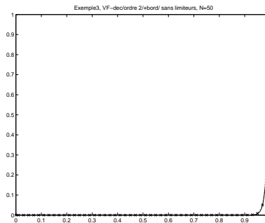
Figure 21: Exemple 3, VF-d/ordre 2/+bord/sans limiteurs, N=50, x=solution approchée
