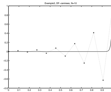
Figure 3: Exemple 3, DF-c, N=10, x =solution approchée
