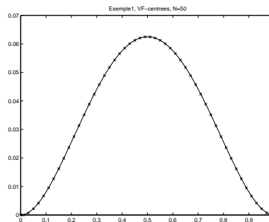
Figure 6: Exemple 1, VF-c, N=50, x=solution approchée
