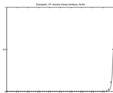
Figure 23: Exemple 3, VF-d/ordre 2/avec limiteurs, N=50, x=solution approchée
