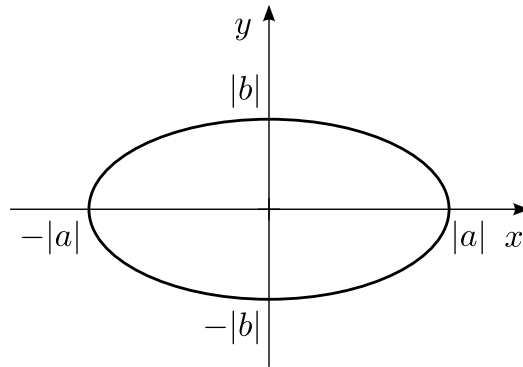
FIG. VIII.1. : Ellipse.
