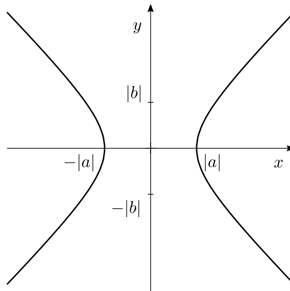
FIG. VIII.2. : Hyperbole.
