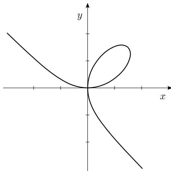
FIG. VIII.3. : Folium de Descartes.
