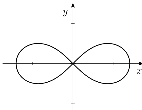
FIG. VIII.4. : Lemniscate de Bernoulli.
