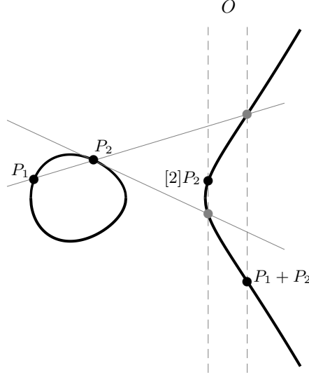
FIGURE 1 – Interprétation géométrique de l'addition sur une courbe elliptique réelle.
