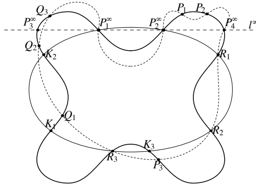
FIGURE 2 – Interprétation de l'addition sur la jacobienne d'une courbe de genre 3 non hyperelliptique.
