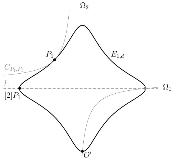
FIGURE 3 – Divers cas de l'interprétation géométrique de l'addition sur une courbe d'Edwards.
