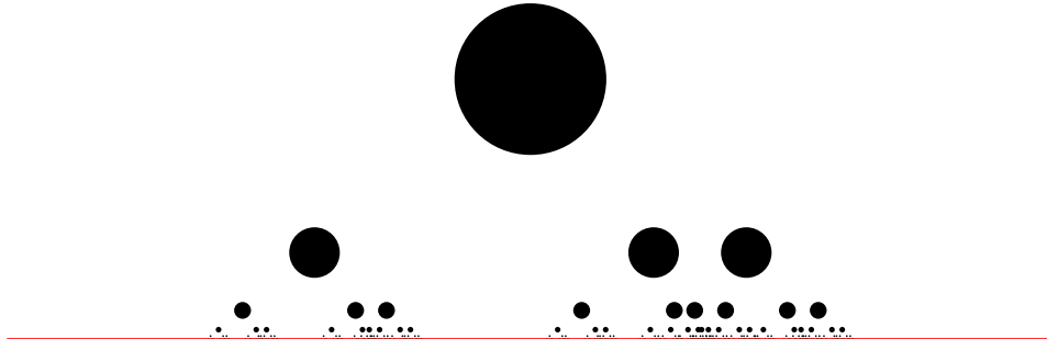
FIGURE II.17 – Développement en base \beta = 3 , avec ensemble de chiffres A = \{0, \frac{\pi}{4}, 1\} .
