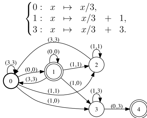
FIGURE III.18 – Automate \mathcal{A}^0 du monoïde engendré par les trois applications
