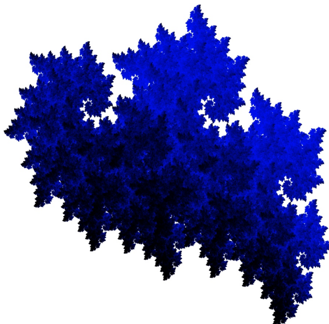
FIGURE I.4 – Ensemble limite d'un sous-semi-groupe de SL(2, \mathbb{C}) agissant par homographie sur la sphère de Riemann \hat{\mathbb{C}} .
