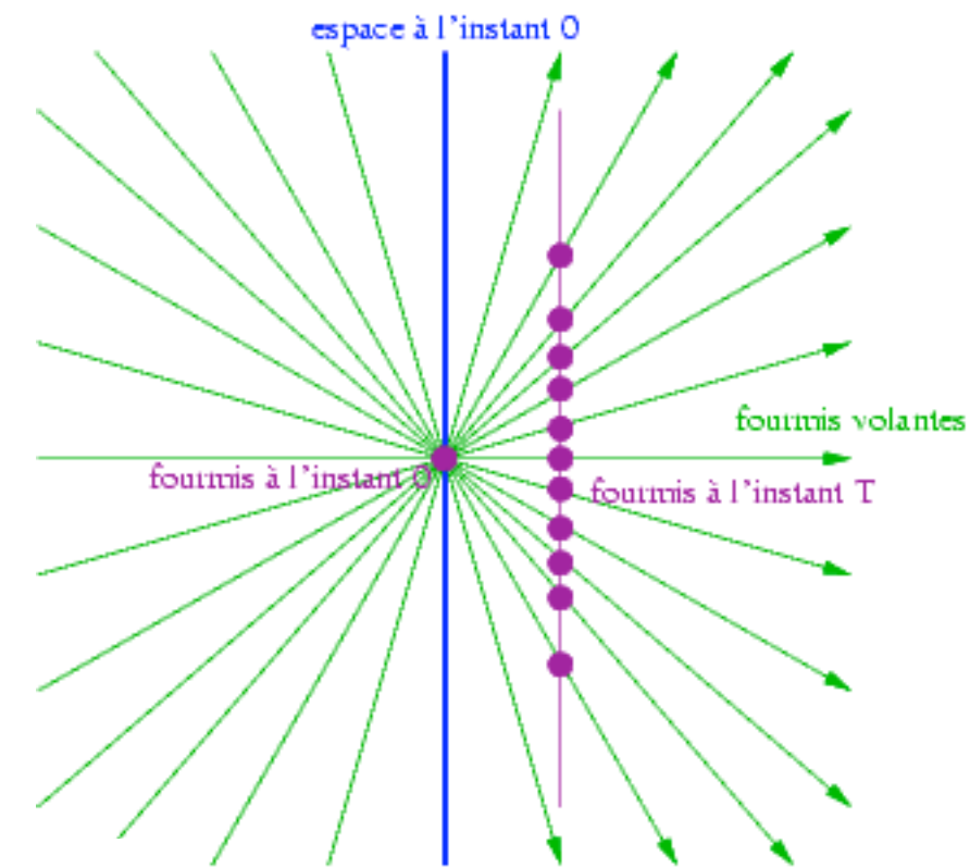
Espace-temps Galiléen
