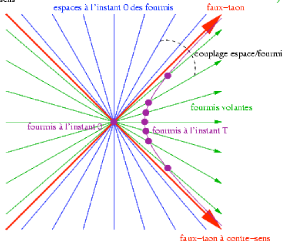
Espace-temps relativiste
