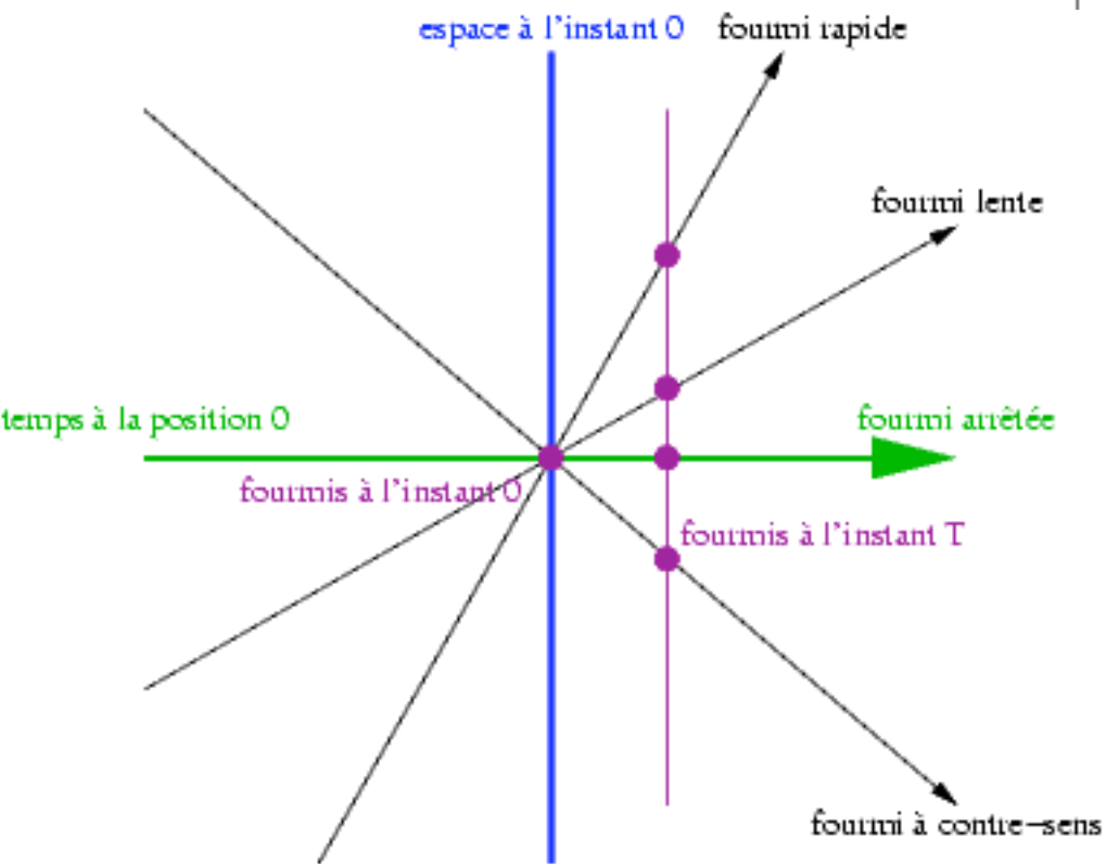
Espace-temps relativiste
